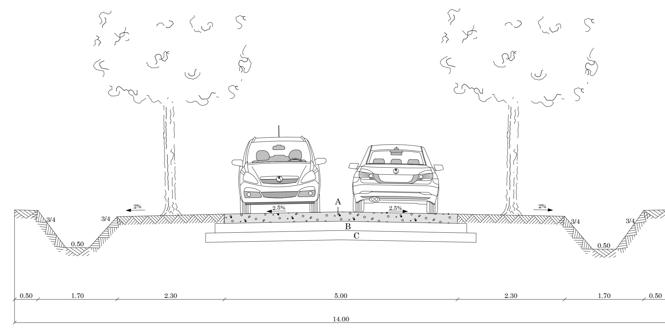
Type-dwarsprofiel A - A' 1/50
