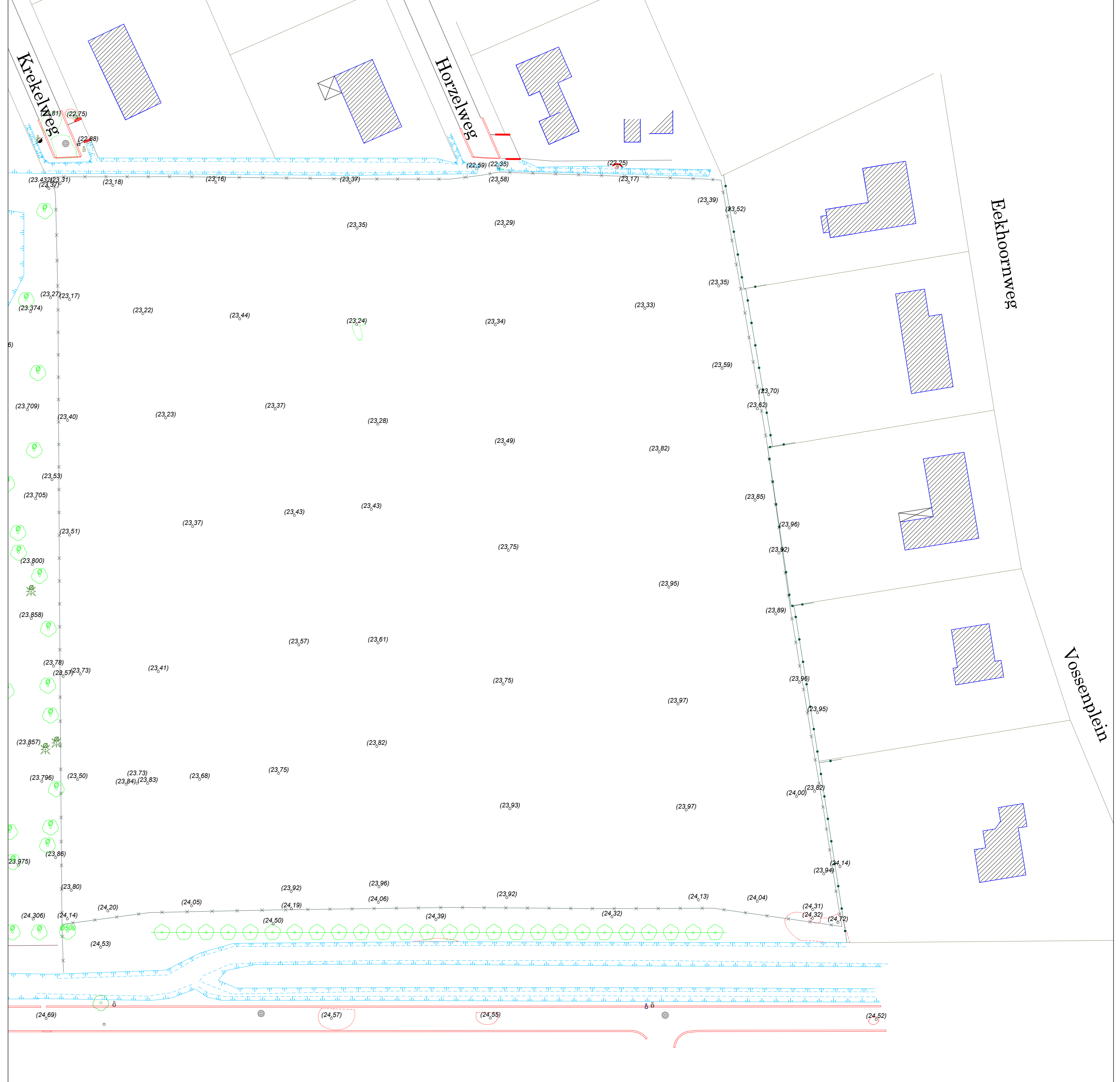
Hoogtes bestaande toestand Schaal 1/500
