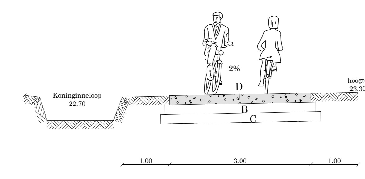
Type-dwarsprofiel B - B' 1/50
