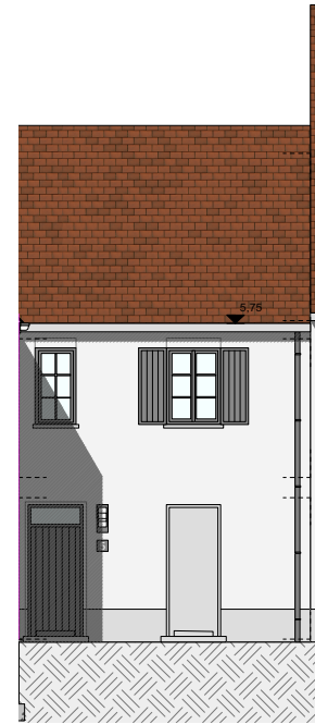
VOORGEVEL
