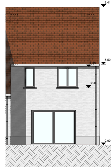
ZIJGEVEL
