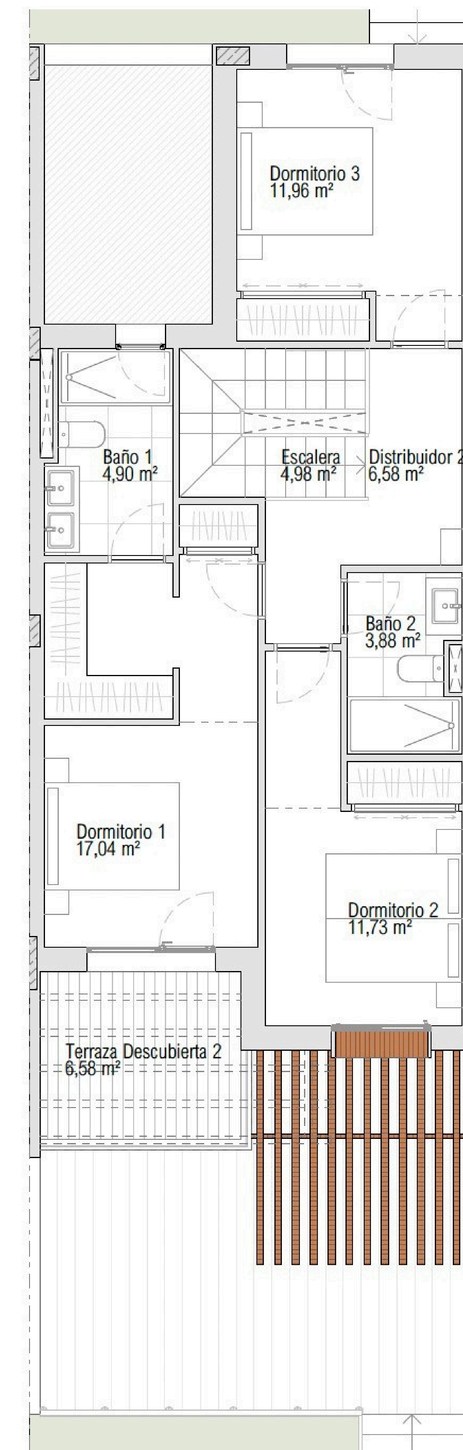
PLANTA ALTA
