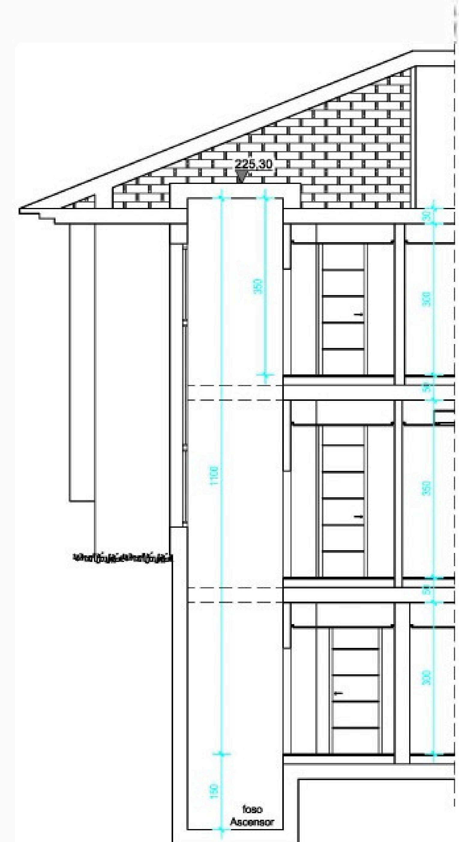
SECCIÓN ASCENSOR
