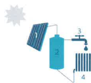
1. Zonnecollector | 2. Opslagvat zonnewater | 3. Sanitair koud water | 4. Aftelcircuit voor ruimteverwarming (opt. afzet)
